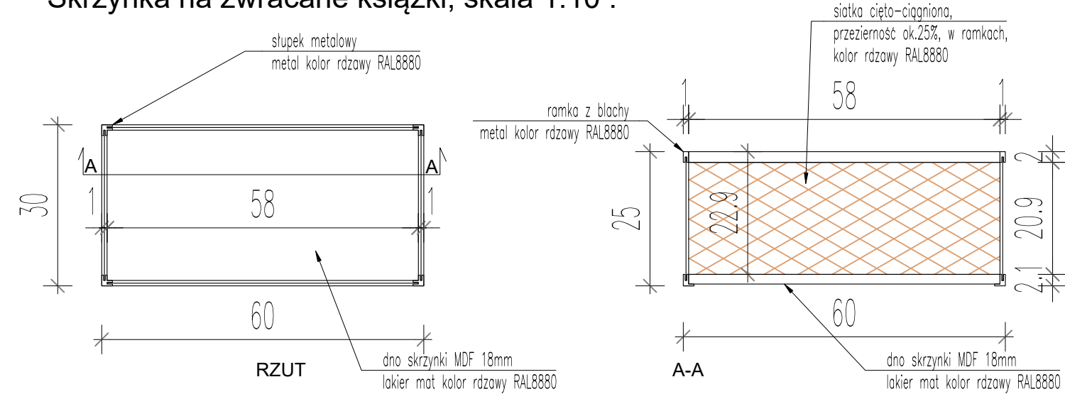
Skrzynka na zwracane książki, skala 1:10 :
