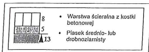
Rys. 3. Przekrój poprzeczny nawierzchni chodnika (wg rozporządzenia Ministra Transportu i Gospodarki Morskiej z dnia 2.02.1999 w spr. warunków technicznych, jakim powinny odpowiadać drogi publiczne i ich usytuowanie, Dz.U. nr 43, poz. 430)
